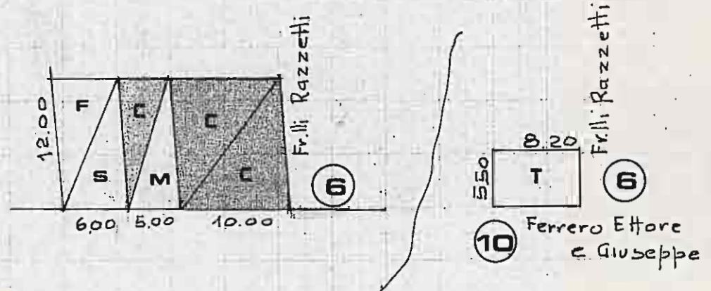
PIANTE
