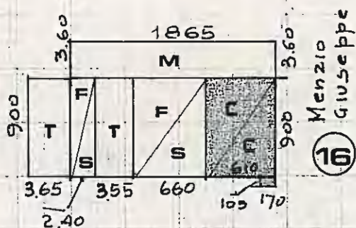
PIANTE
