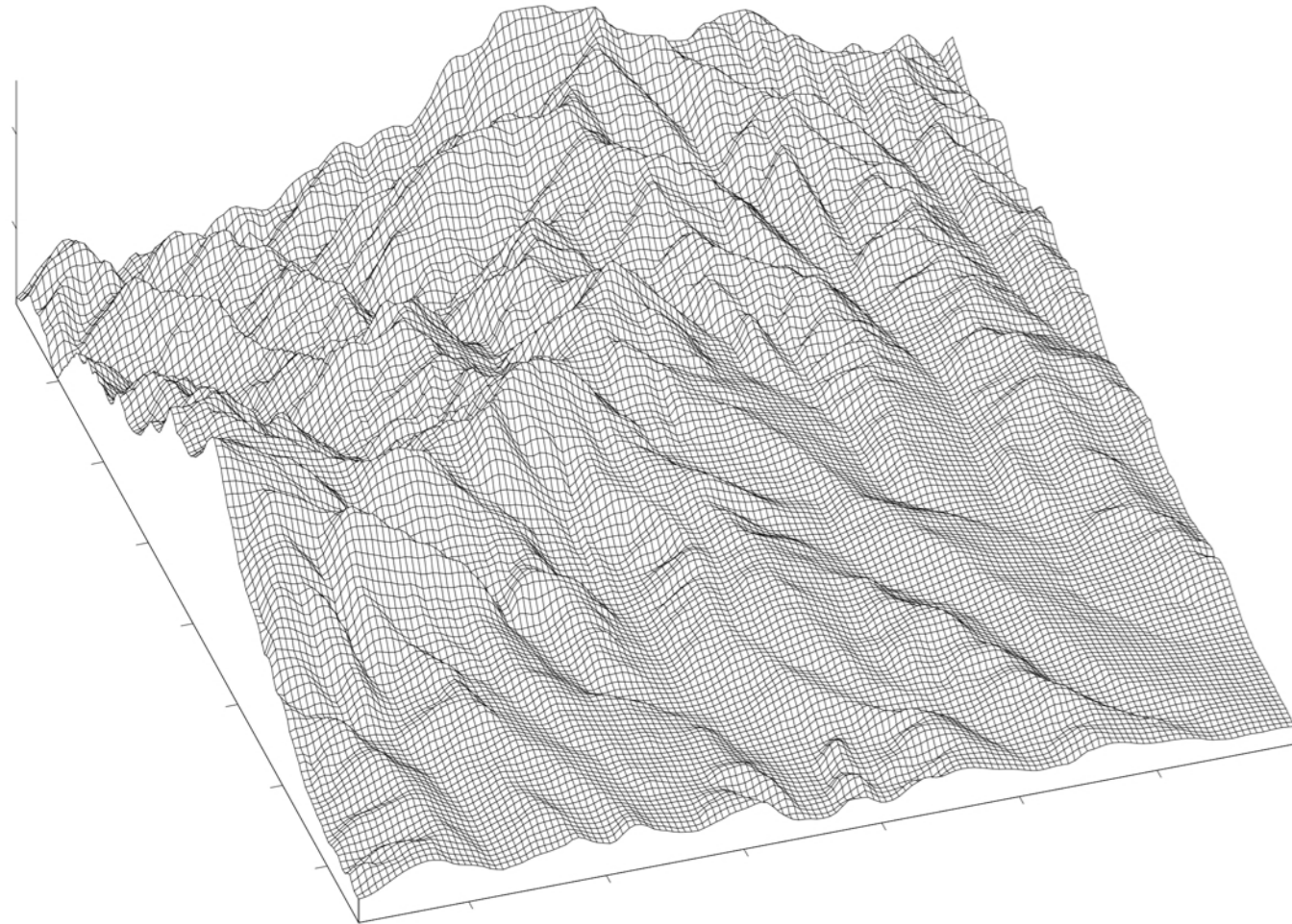
Modello altimetrico digitale dal DTM della Regione Piemonte (vista da S-SE, vert. 4x)
